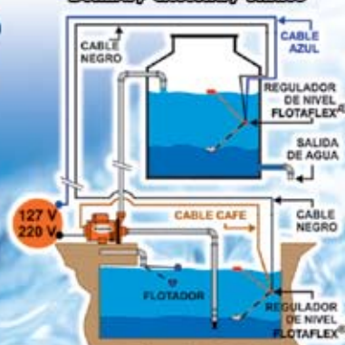
INSTALACIÓN TIPO B Bomba / Tinaco
